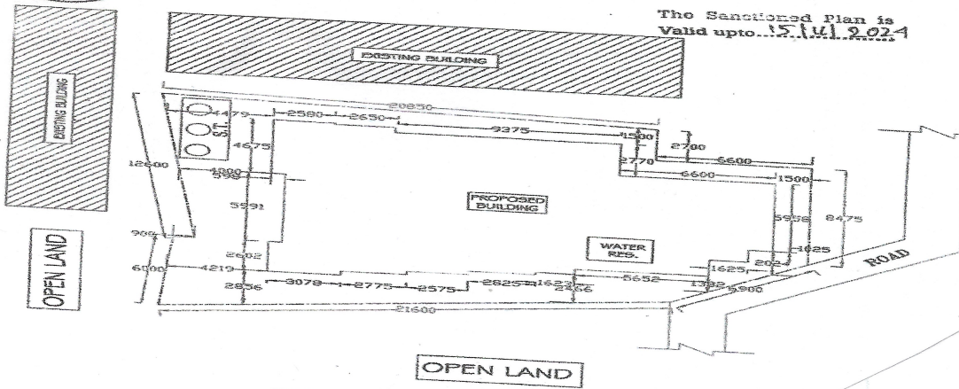
SITE PLAN (SCALE :- 1:200)
