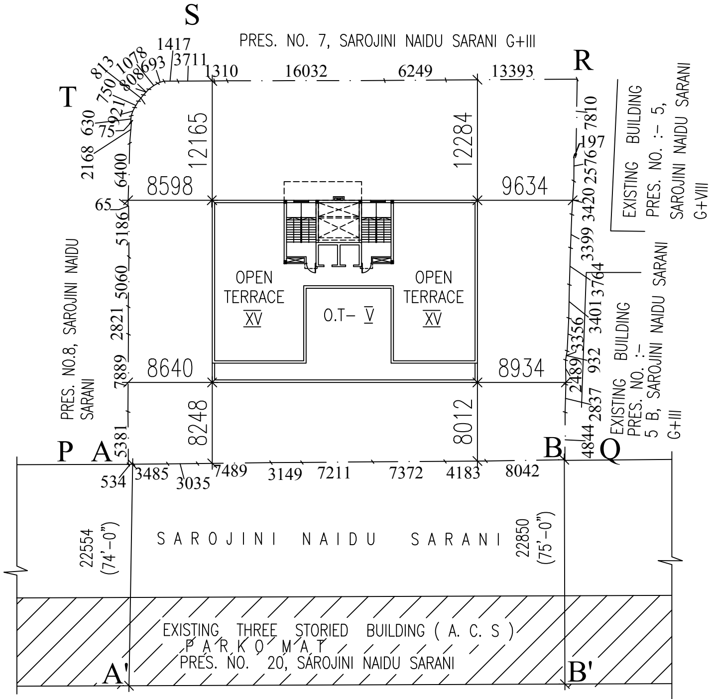
SITE PLAN SCALE-1:600
