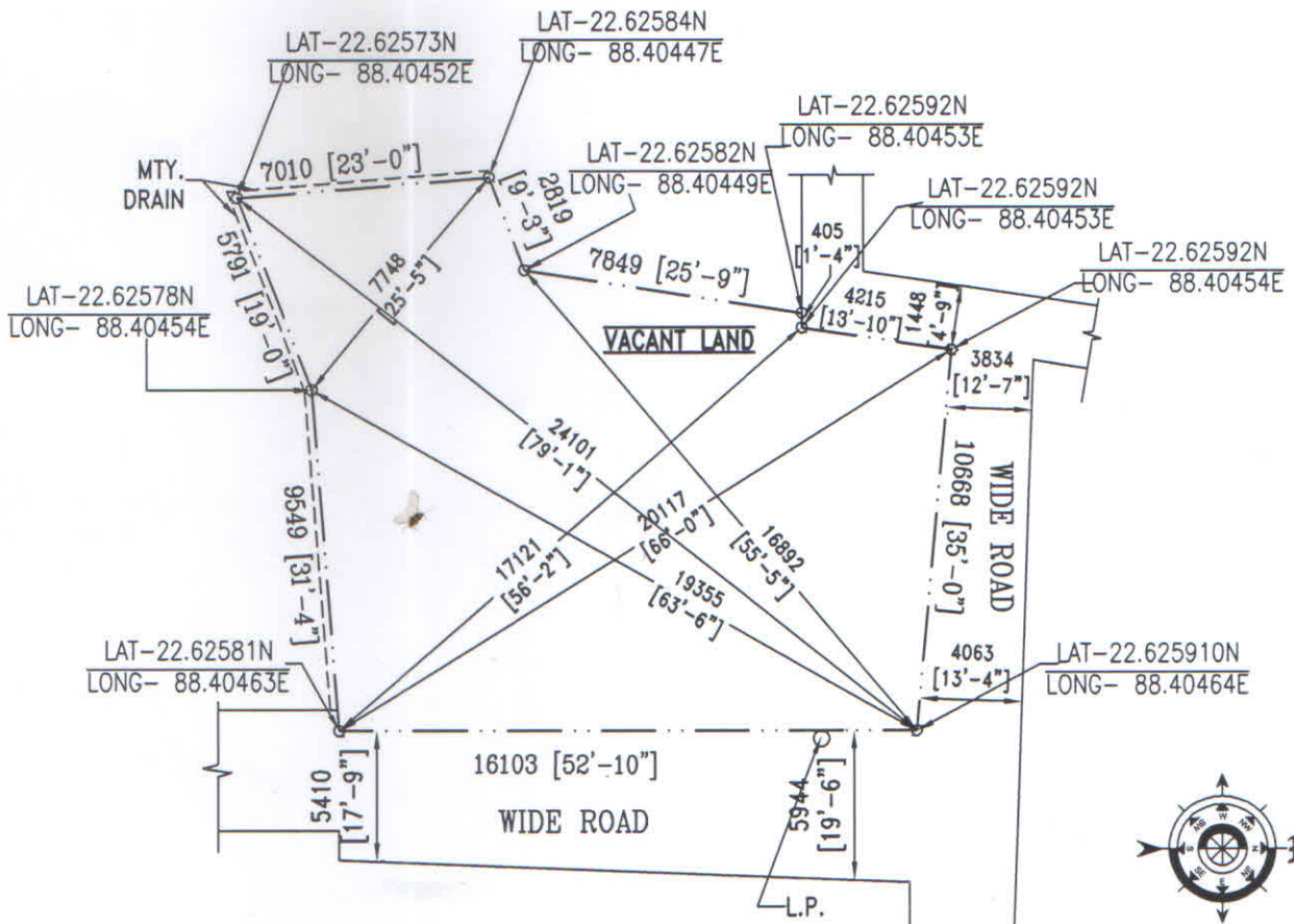
LATITUDE & LONGITUDE PLAN SCALE = 1:200
