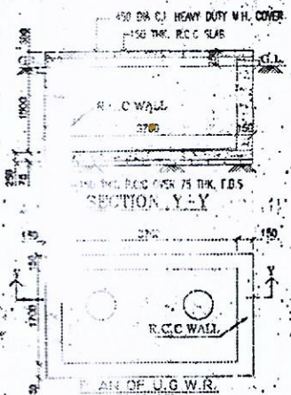
PLAN OF U.G.W.R. SCALE: 1:50
