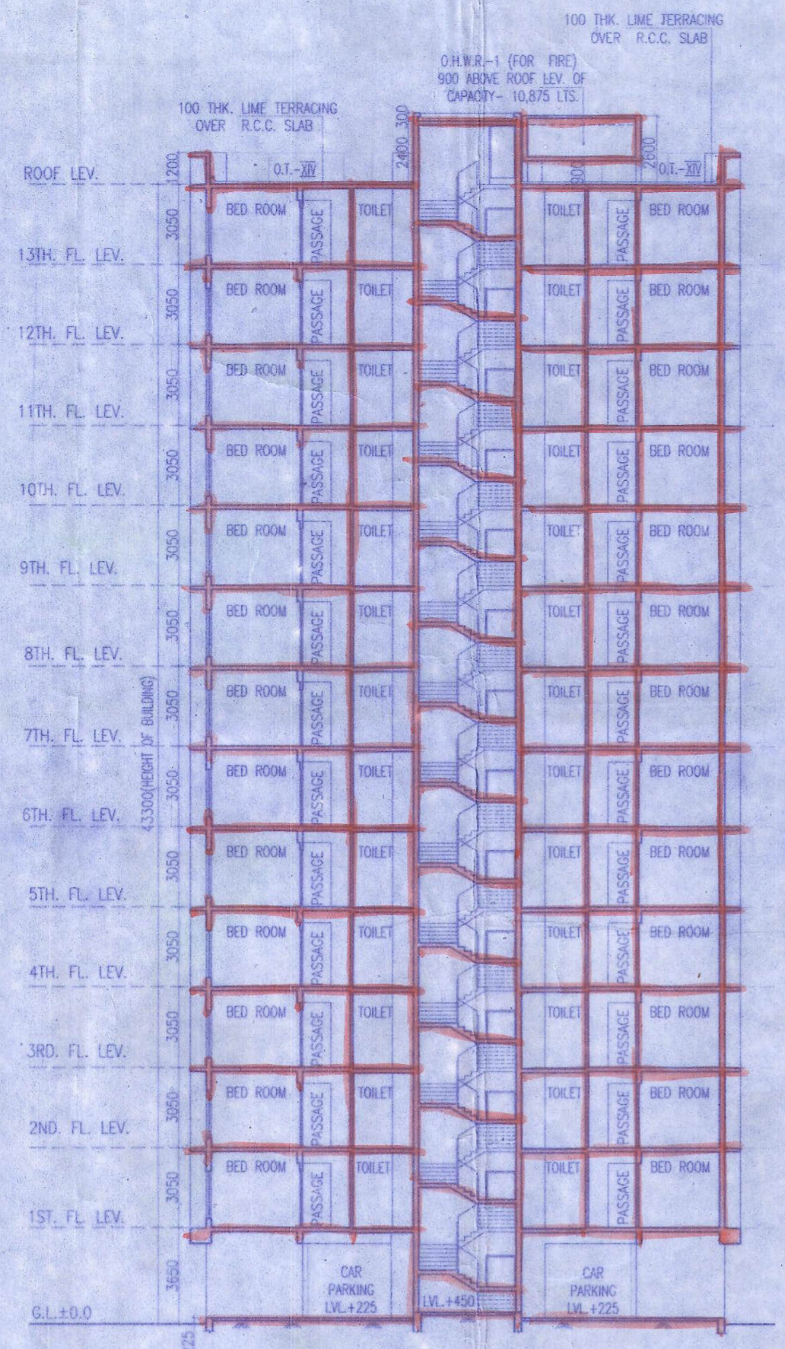
SECTION : A7 - A7
