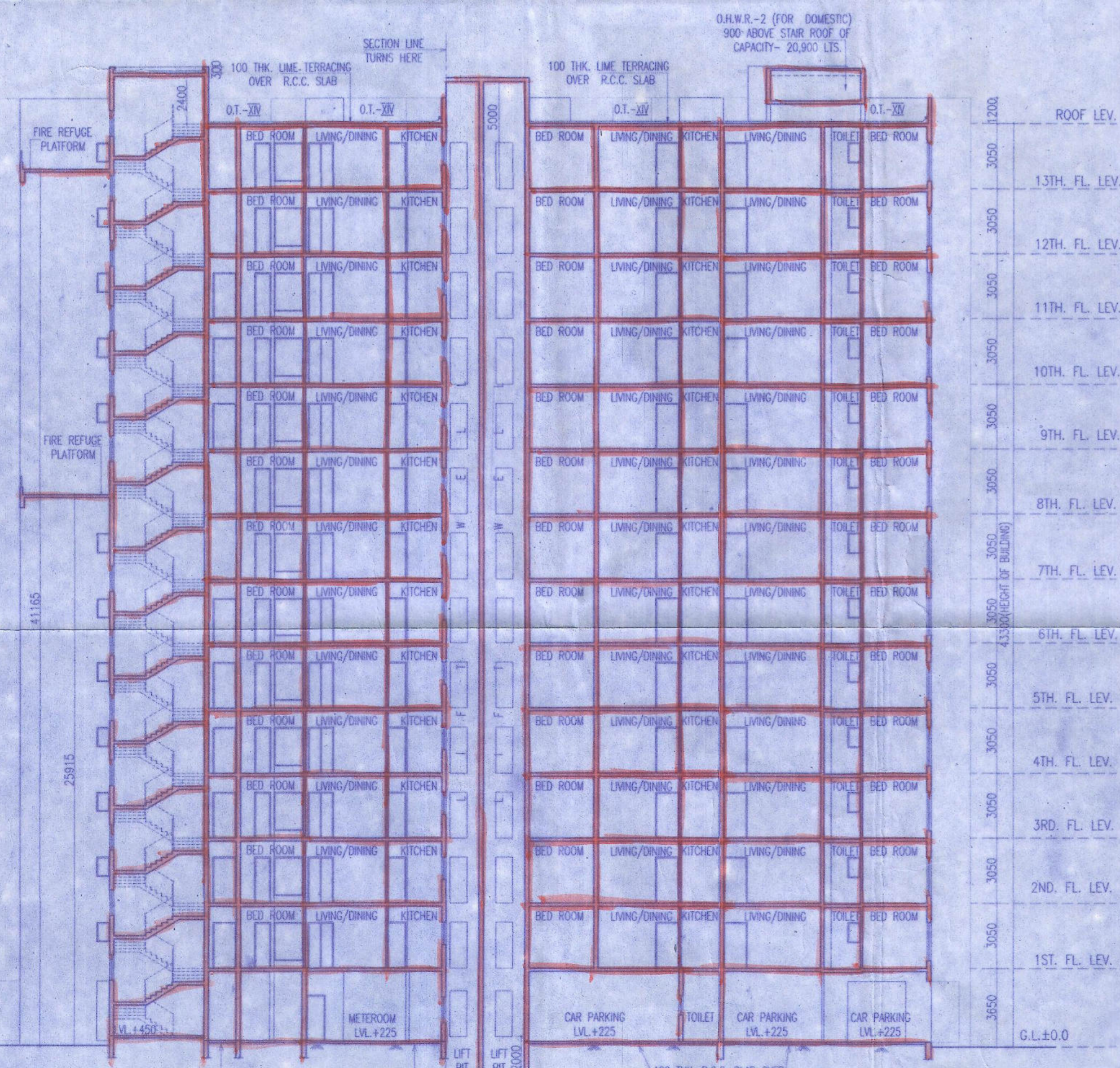
SECTION : A8 - A8
