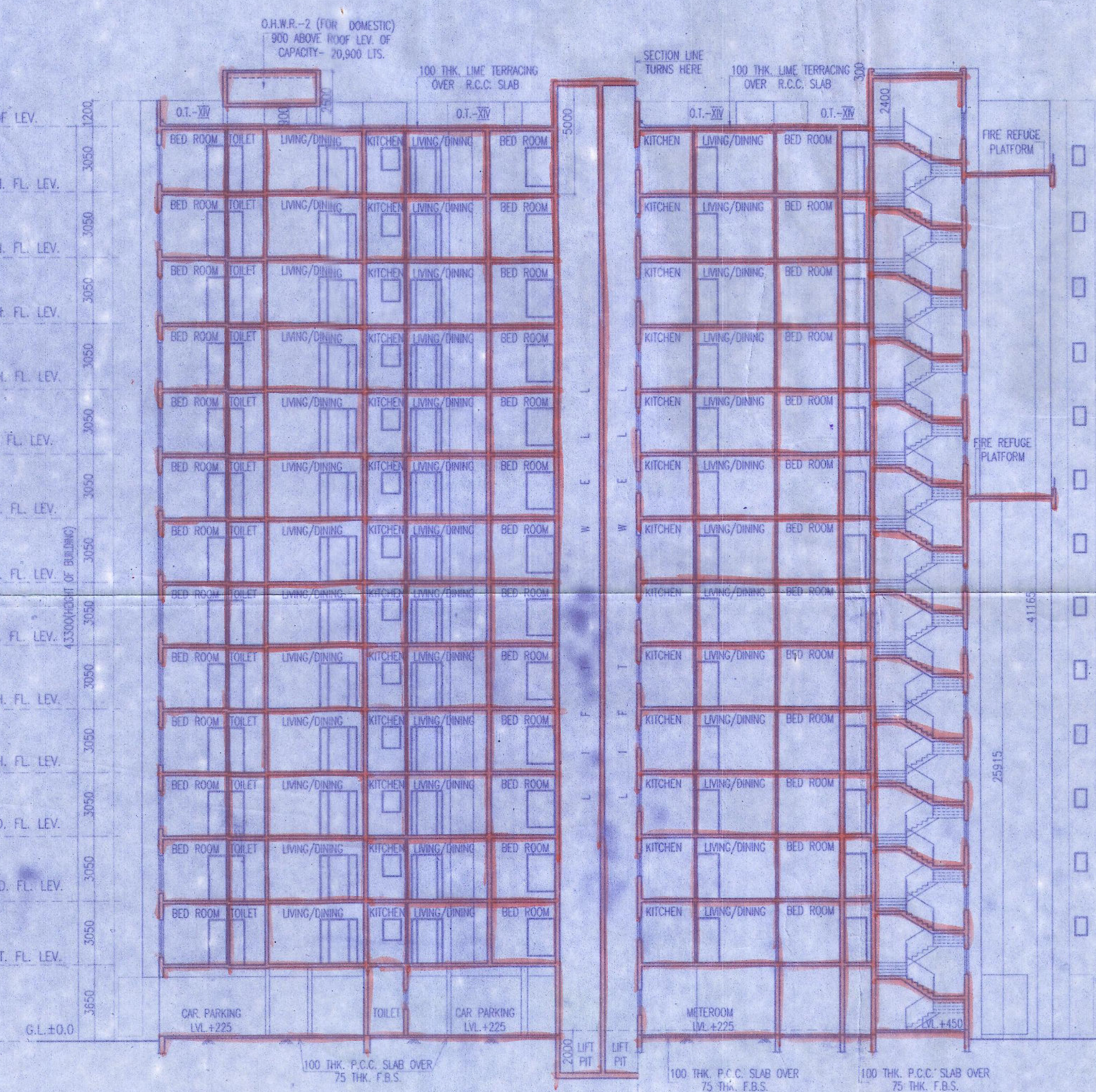
FRONT ELEVATION SECTION : A2 - A2
