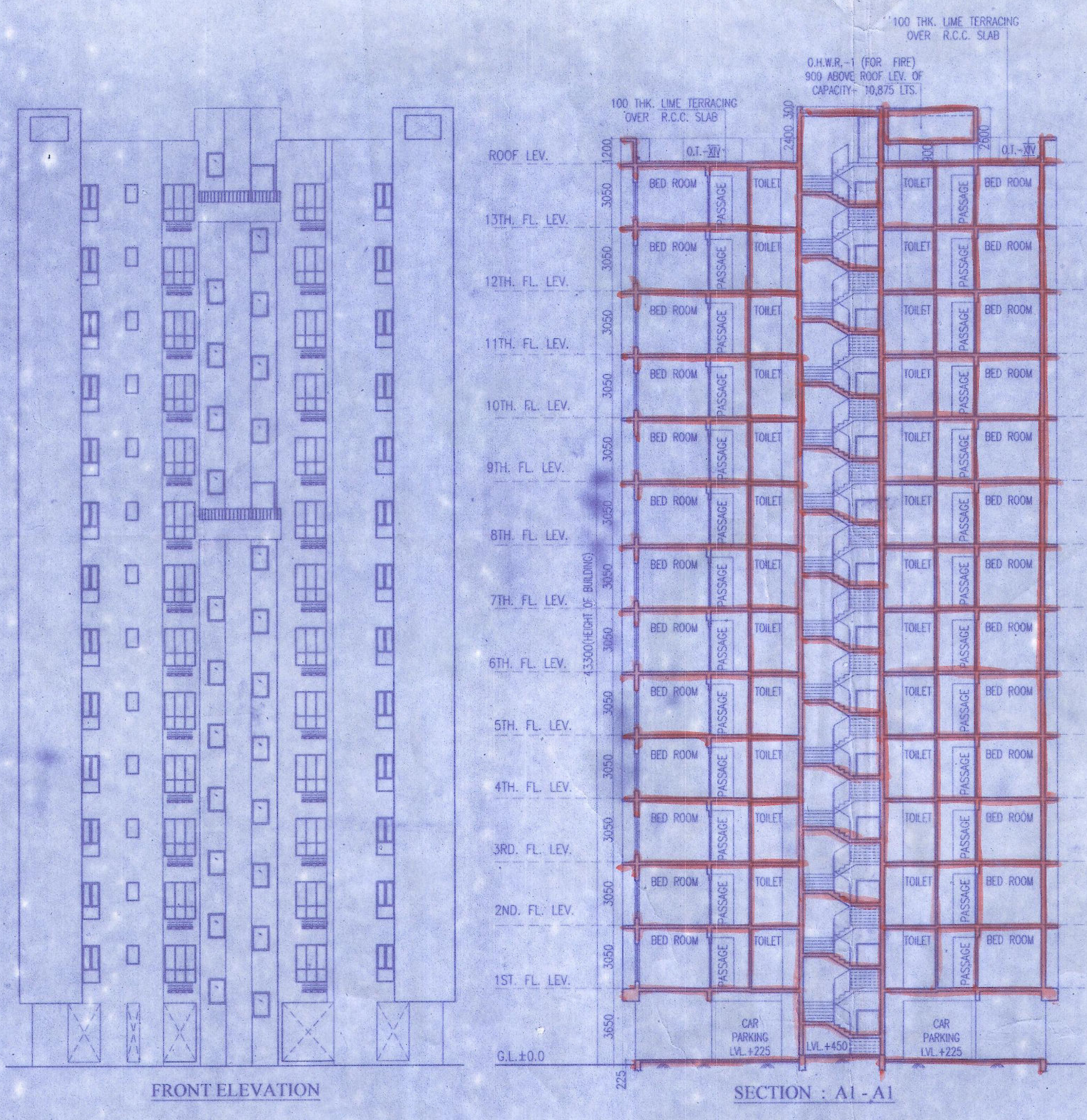
FRONT ELEVATION SECTION : A1 - A1
