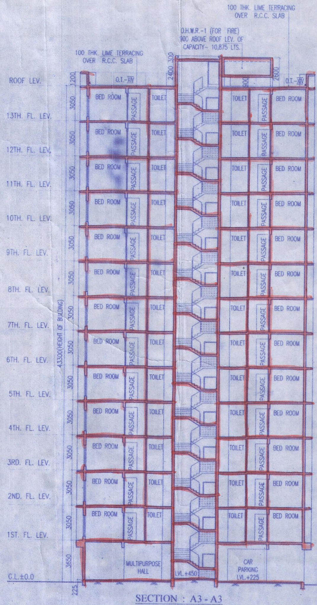
SECTION : A3 - A3
