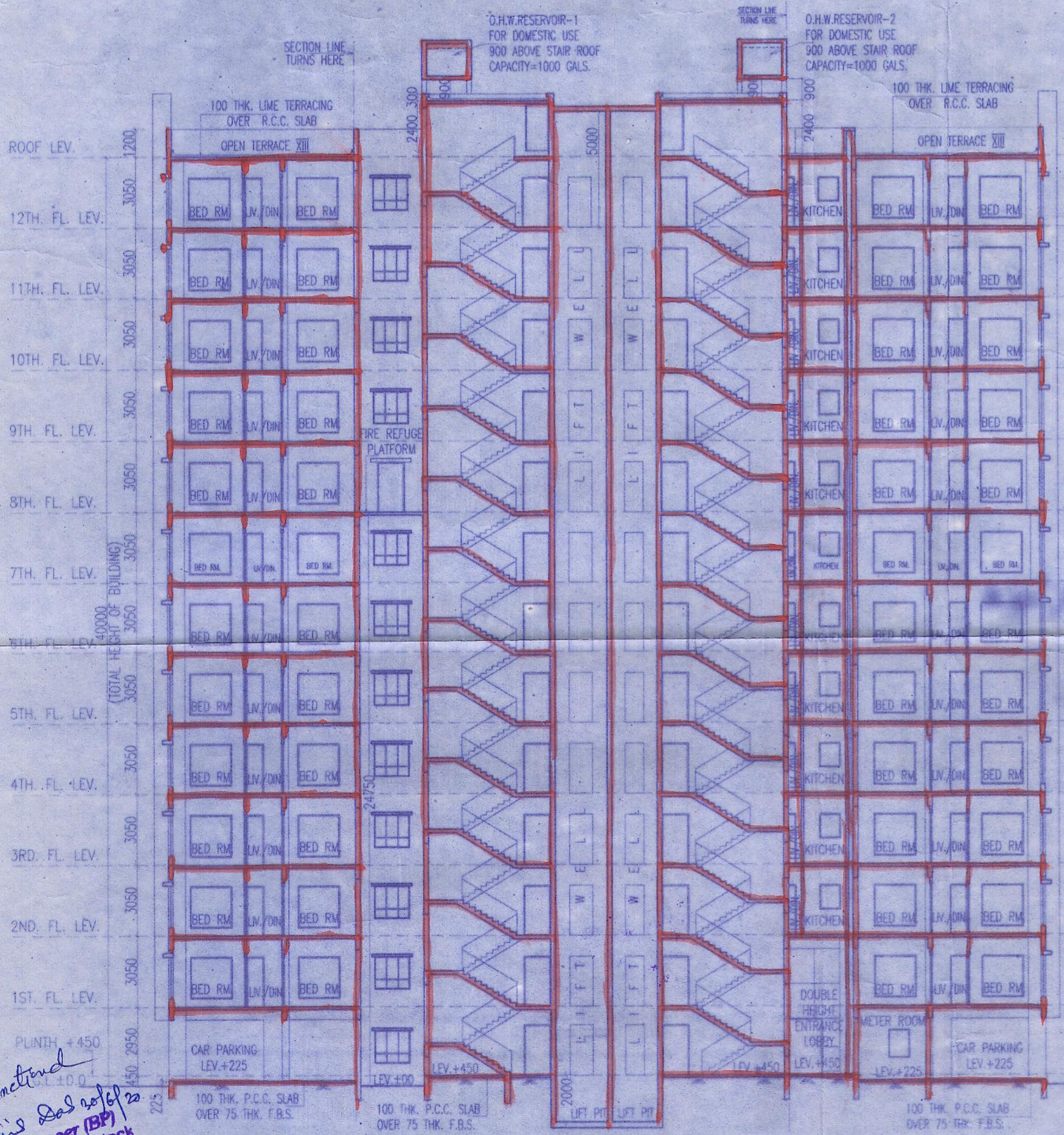
SECTION - F4 - F4
