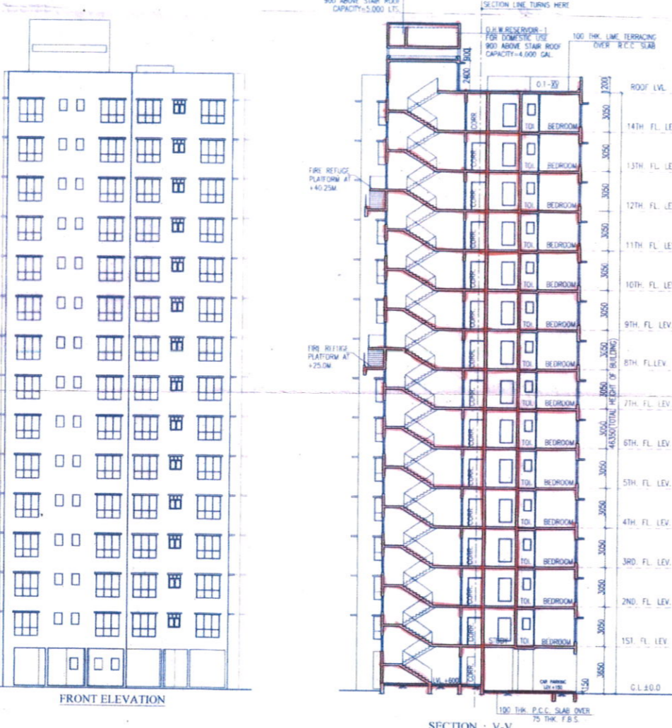
SECTION - V-V
