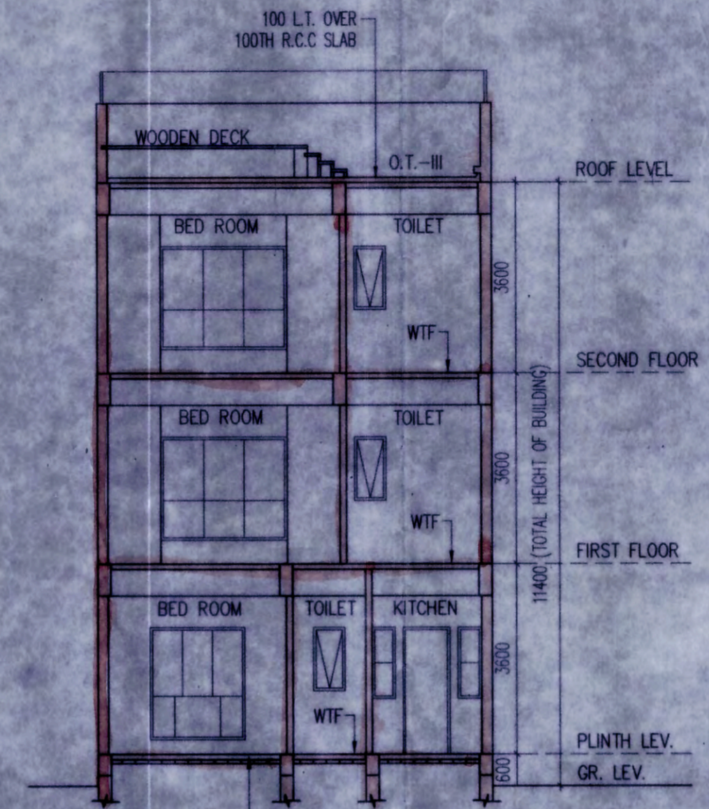
SECTION D-D
