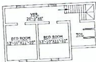
Ist FLOOR PLAN PROPERTY AMAR BHATTACHERJEE
