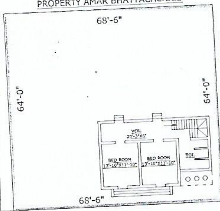
Ist FLOOR PLAN PROPERTY AMAR BHATTACHERJEE
