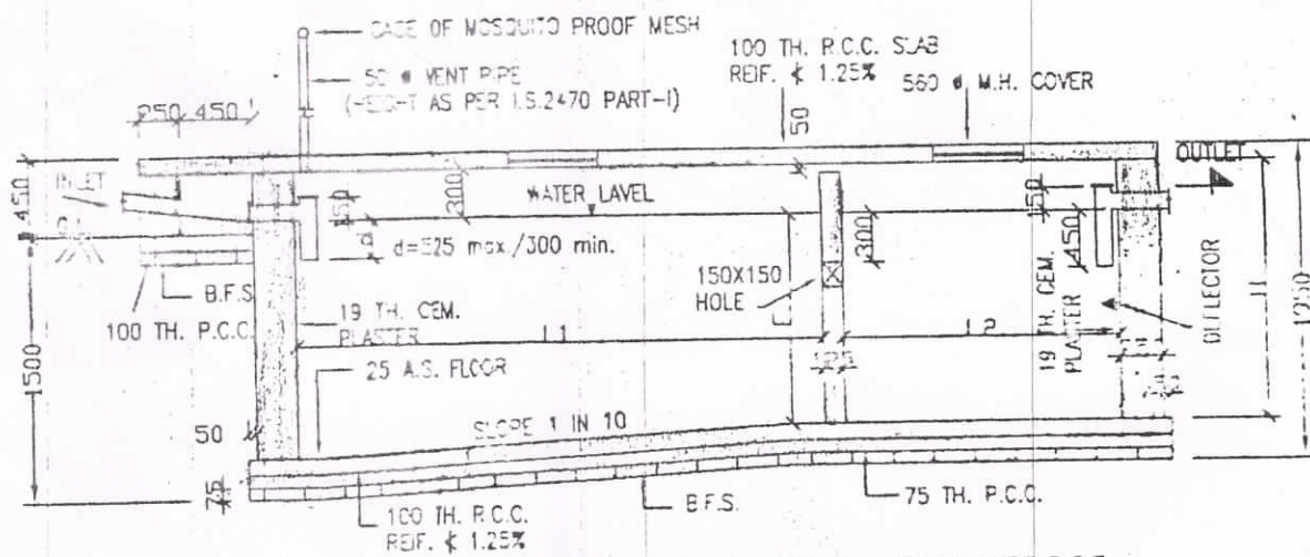
LONGITUDINAL SECTION
